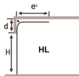
Paaukštintas pakilimas
