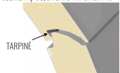
SEGMENTŲ SUJUNGIMO FRAGMENTAS
